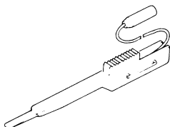
453718 BERG MINIPROBE 453705 BERG LATCH UNLATCH TOOL
